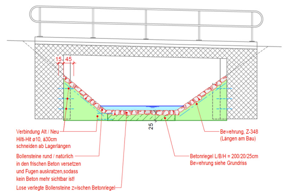
Querschnitt 1-1 1:50
